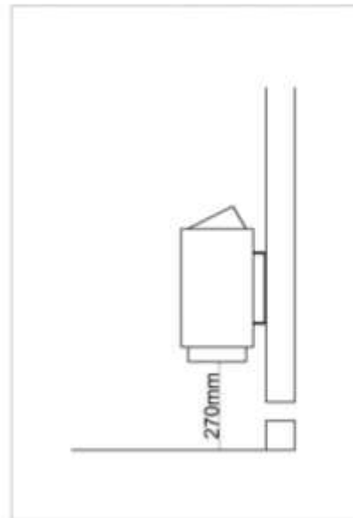
Resim 4: SAUNA ISITICISI - ZEMİN ARASI MONTAJ
