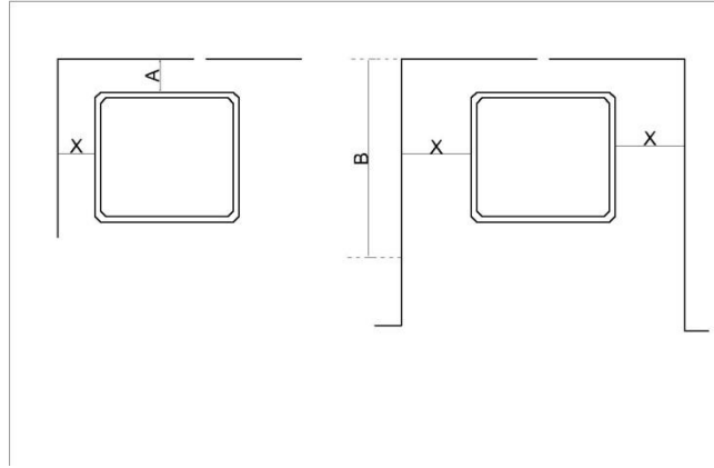
Resim 2: ASGARİ EMNİYETLİ MONTAJ MESAFELERİ - Tablo 2'ye bakınız.
